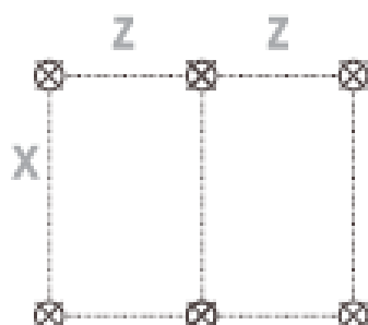
Diagrama de anclajes para baterías de dos y de más de dos colectores (hasta 5)
