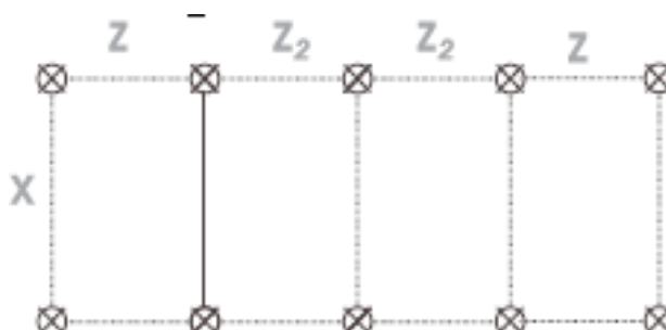
Diagrama de anclajes para baterías de dos y de más de dos colectores (hasta 5)
